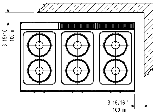
Felülnézet
