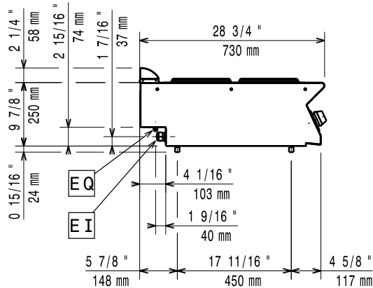
Oldalnézet
